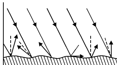
Fig. : Diffused reflection
